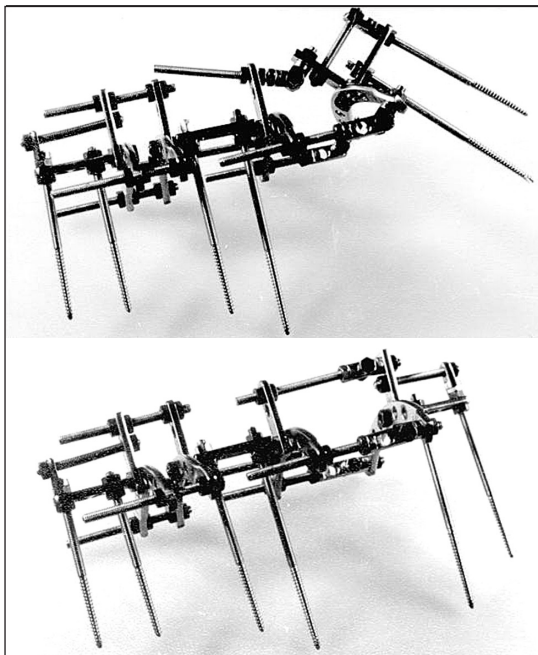
Рис. 12. Фото разработанных в институте аппаратов внешней фиксации на стержневой основе
