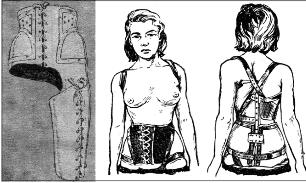
Рис. 10. Разработанные в институте облегченный аппарат и корригирующий корсет
