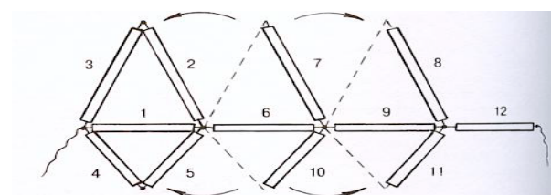
Схема модуля павука-зірки
