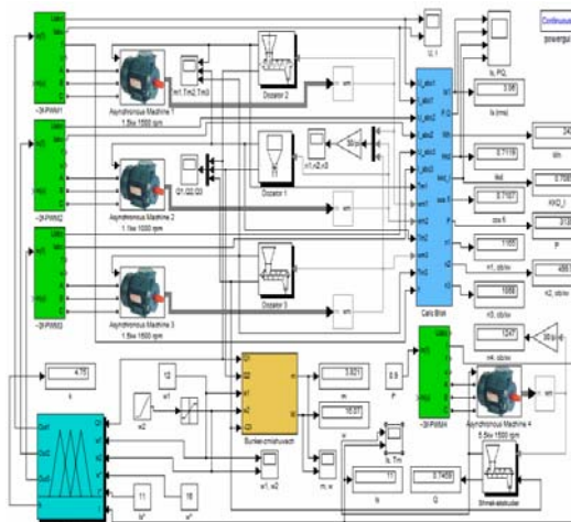
Рис. 1. Імітаційна модель установки для виробництва двокомпонентного твердого біопалива
