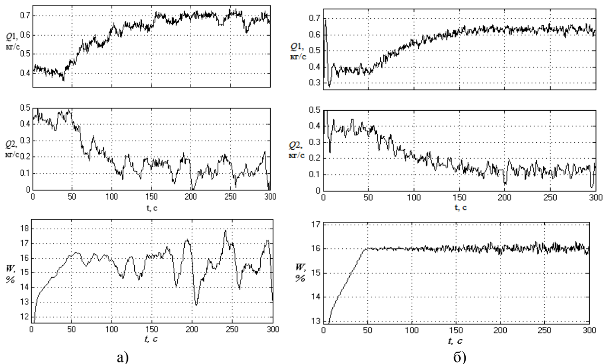
Рис. 3. Дисперсії продуктивностей дозаторів Q_1, Q_2 та вологості суміші w : а) – без корекції, б) – з корекцією швидкостей робочих органів дозаторів
