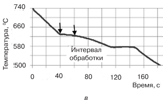
Рис. 1. Температурно-временной интервал МИО: а – y = 20 ; б – y = 10 ; в – y = 5
