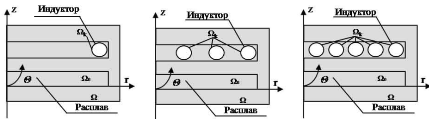
Рис. 5. Геометрическая модель МИО
