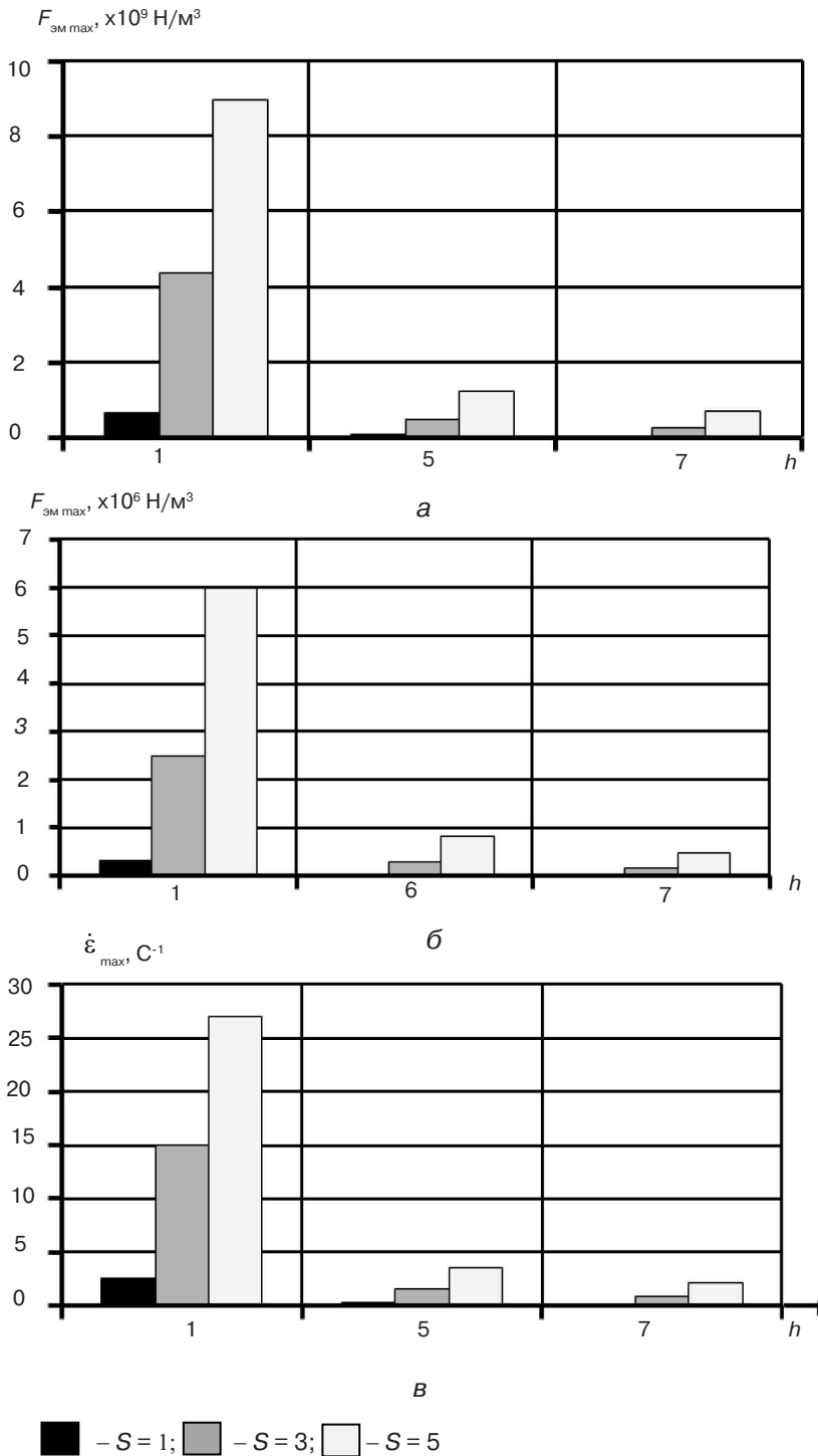
Рис. 6. Параметры МИО в момент времени, соответствующий первому максимуму разрядного тока, в зависимости от высоты размещения индуктора над поверхностью и количества витков: а – объемная электромагнитная сила; б – магнитное давление; в – скорость деформации
