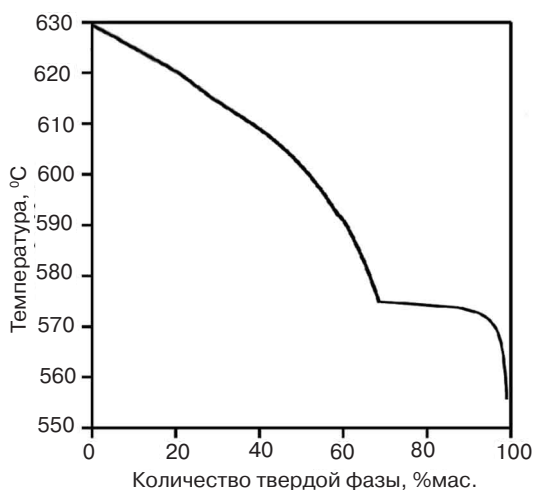
Рис. 2. Изменение доли твердой фазы в сплаве А357
