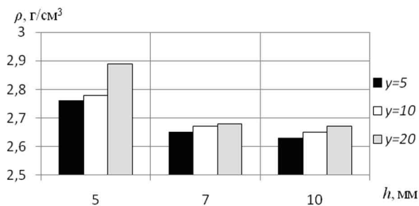
Рис. 4. Изменение плотности сплава А357 при МИО (плотность необработанного сплава – 2,63 \text{ г/см}^3 )
