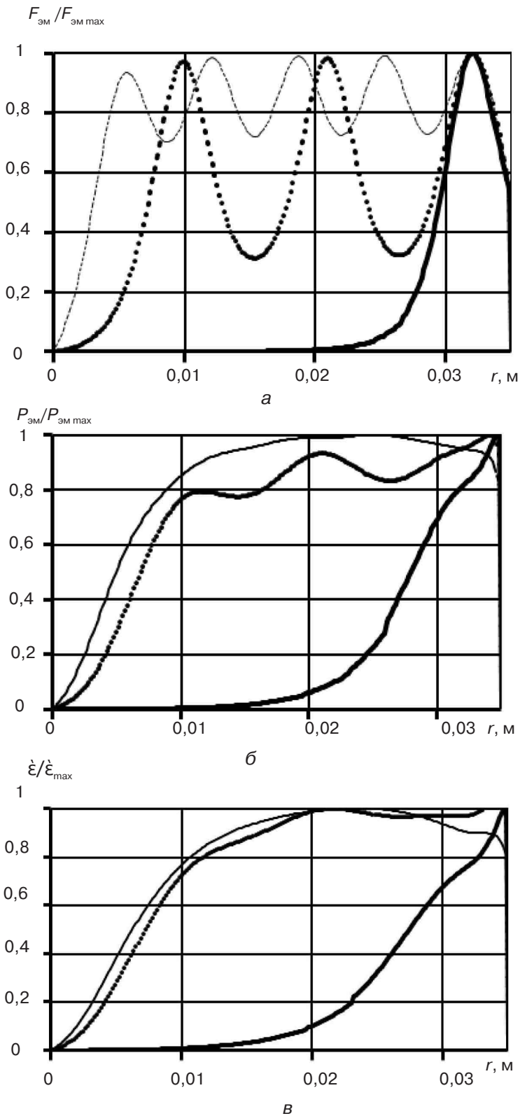
Рис. 7. Распределение параметров МИО по радиусу слитка в зависимости от количества витков индуктора: а – относительная объемная электромагнитная сила; б – относительное магнитное давление; в – относительная скорость деформации
