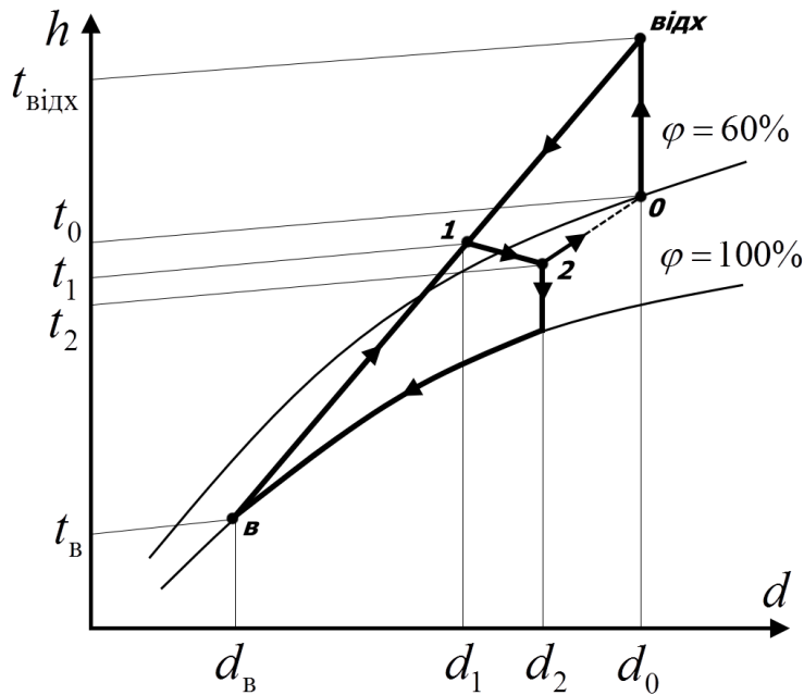
Рис. 2. Процес тепловологообробки повітря в системі кондиціонування плавального басейну з частковою рециркуляцією.
