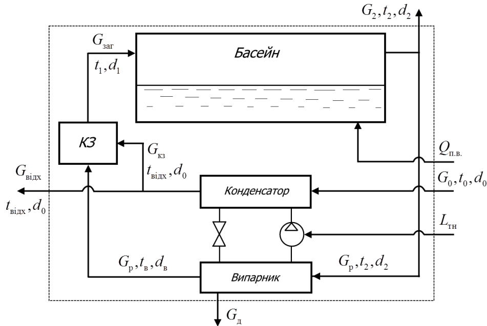
Рис. 1. Принципова схема кондиціонування повітря плавального басейну з частковою рециркуляцією: КЗ – камера змішування.
