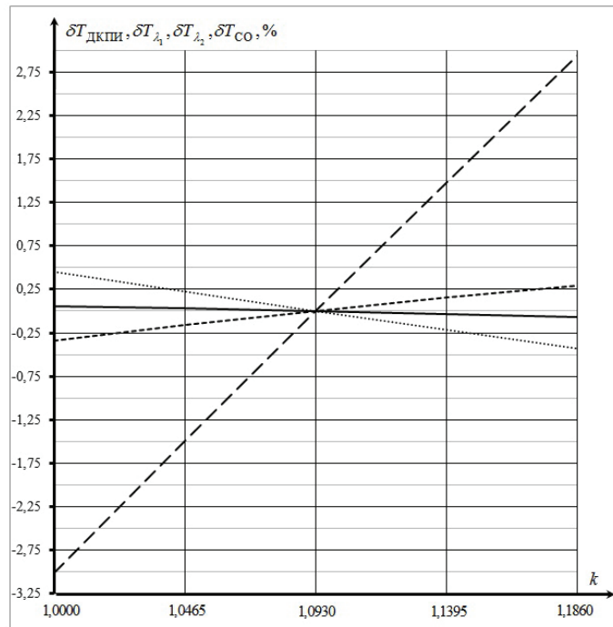
Рис. 2. Влияние селективности излучения металлических сплавов на относительные методические погрешности пирометрии излучения при T = const = 1600\text{K} и \varepsilon_{cp} = const = 0,417 :
