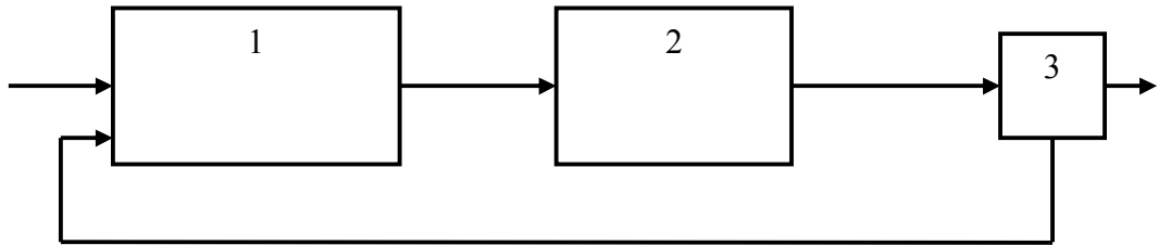
Рис. 2. Метод біологічного видалення фосфору A/O (Anaerobic-Oxic): 1 – анаеробна зона; 2 – аеробна зона; 3 – вторинний відстійник
