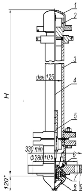
Рис.1. Схема улаштування пожежного гідранту підземного типу: 1 – кришка (поліетилен); 2 – ніпель (бронза); 3 – корпус (сталь); 4 – штанга (сталь); 5 – шпindel (нержавіюча сталь); 6 – коропус клапана (бронза); 7 – кільце; 8 – гайка клапана (чавун); 9 – патрубок (чавун)
