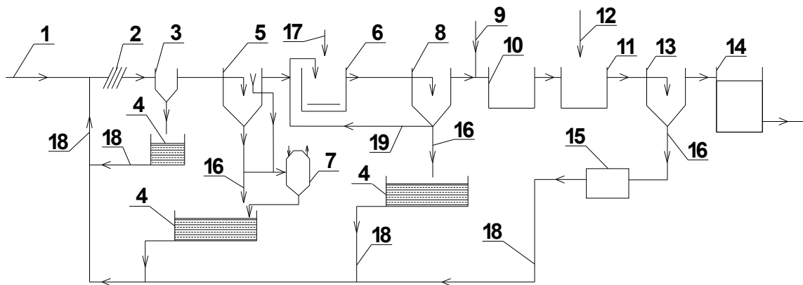
Рис. 1. Загальна технологічна схема очищення господарсько-побутових стічних вод: 1 – подача вихідної стічної води; 2 – решітки; 3 – пісковловлювач; 4 – мулові майданчики; 5 – первинний відстійник; 6 – біофільтр або аеротенк; 7 – метантенк; 8 – вторинний відстійник; 9 – подача хлору; 10 – контактний резервуар; 11 – місткість для коагуляції; 12 – подача реагентів; 13 – відстійник; 14 – піщаний фільтр; 15 – згущувач осаду; 16 – скидання осаду; 17 – подача повітря; 18 – відведення відстоюної води; 19 – відведення надлишкового активного мулу в аеротенк
