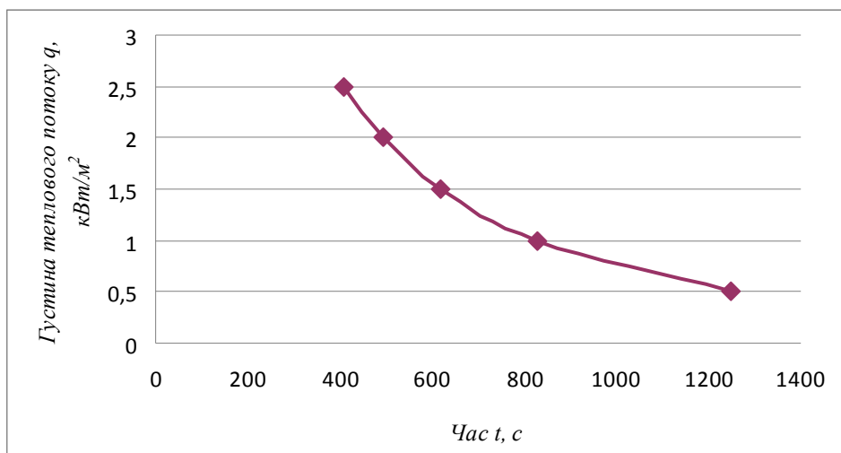
Рис. 2. Значення граничного часу перебування пожежника в ТЗОП від дії НТФ пожежі
