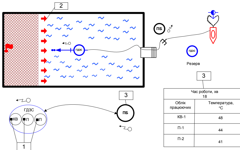
Рис. 3. Схема застосування приладу під час гасіння пожежі:
