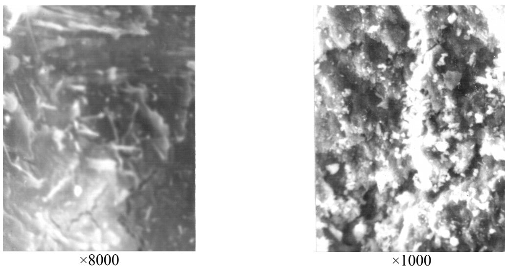
Рис. 2. Мікроструктура каменю на основі портландцементу ПЦ І-500, гідратованого 7 діб
