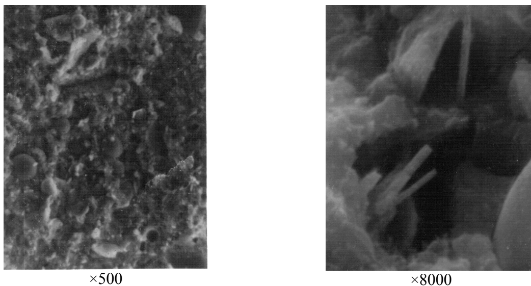
Рис. 3. Мікроструктура каменю на основі портландцементу з додатком золи-виносу, гідратованого 7 діб
