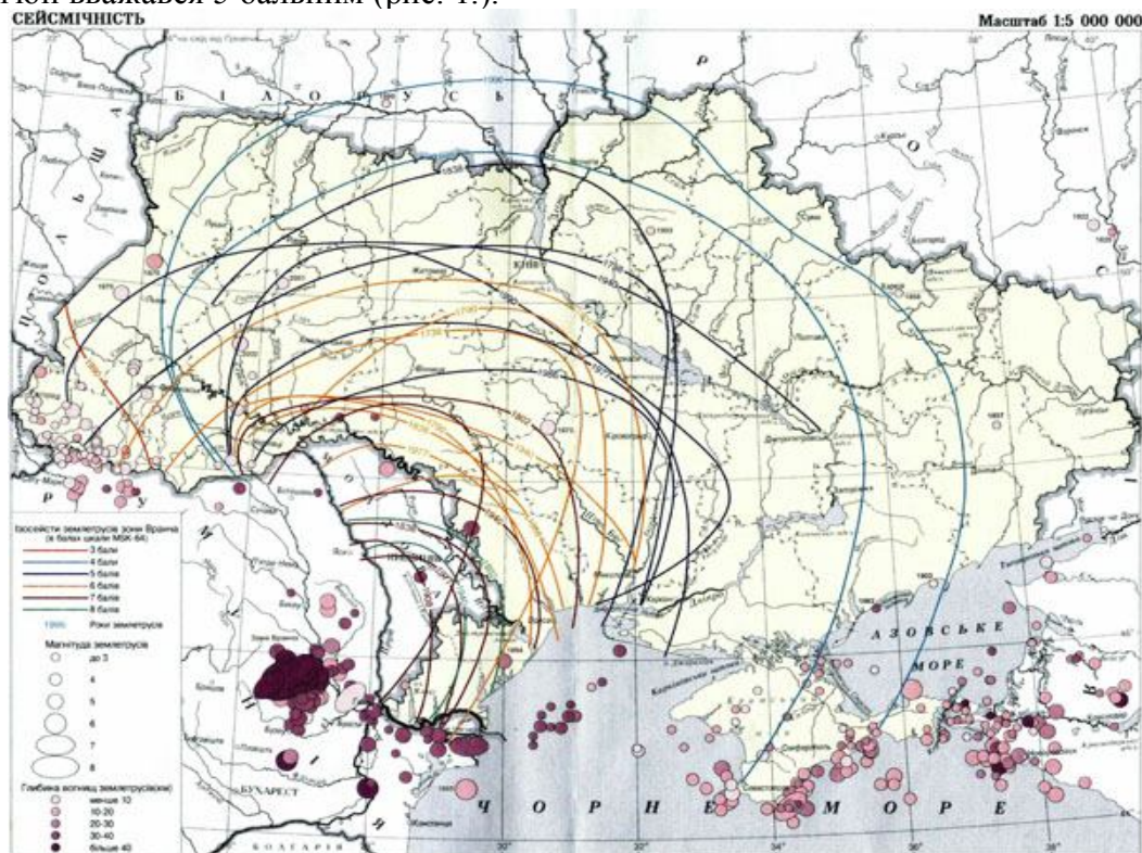
Рис. 1. Карта сейсмічності території України (Автори: Кендзера О.В., Пустовітенко Б.Г., Кутас В.В., Кульчицький В.Є., Вербицький С.Т., Пронишин Р.С., Сафронов О.М., Корольов В.О., Калітова І.А., Пасинков Г.Д., Стасюк А.Ф.) [4]
