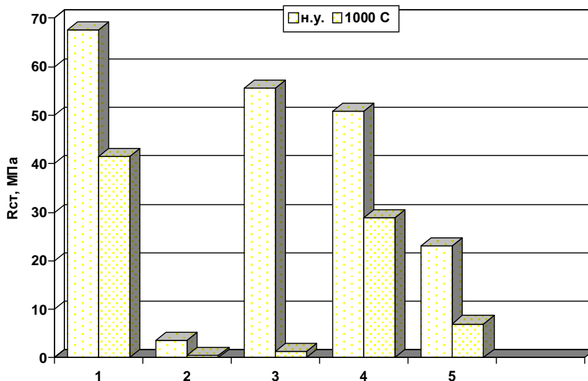
Рис. 1. Міцність цементних мінералів у віці 28 діб при нагріванні до 1200 0 С: 1 – C 3 S, 2 – β-C 2 S, 3 – C 4 AF, 4 – CA, 5 – C 12 A 7
