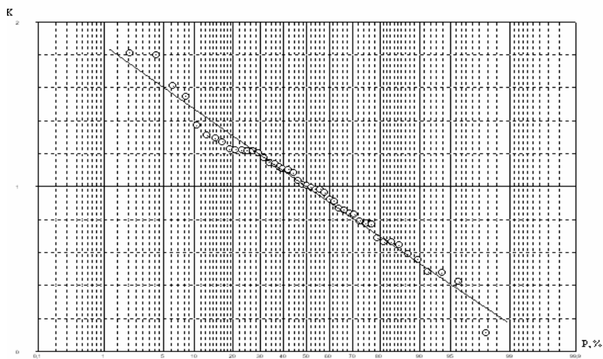
Рис.3. Крива забезпеченості стоку р. Сіверський Донець – м. Зміїв
