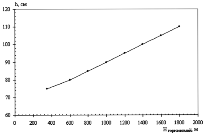
Рис. 2. Залежність ізотерм максимальних глибин промерзання ґрунту від висот горизонталей на топографічній карті для гірської території Чернівецької області
