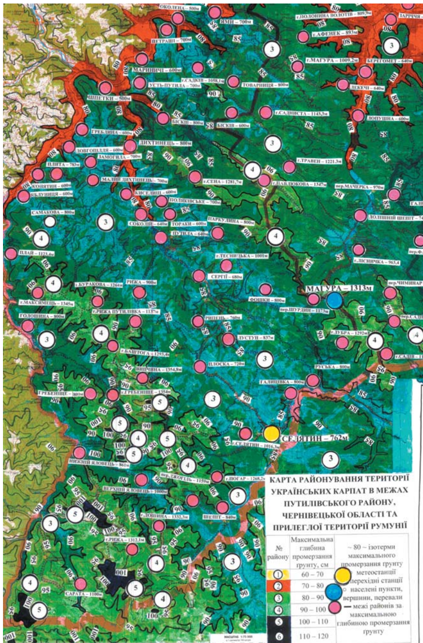
Рис. 3. Карта районування території Українських Карпат у межах Путилівського району Чернівецької області та прилеглої території Румунії за максимальною глибиною промерзання ґрунту
