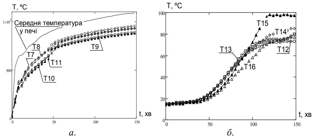
Рисунок 4 – Результати вимірювань температур у зразку №1: на обігрівній поверхні (а) та на необігрівній поверхні (б).
