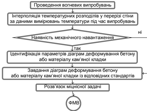
Рисунок. 1 – Схема здійснення оцінки вогнестійкості за допомогою інтерпретації результатів вогневих випробувань залізобетонних несучих стін.
