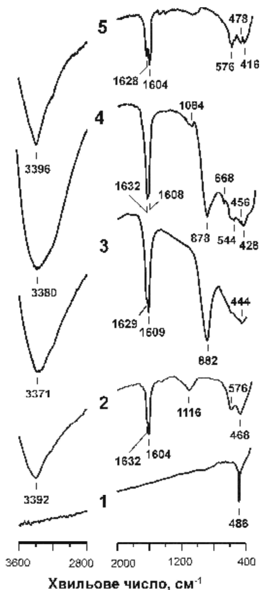
Рис. 5. ІЧ спектри TiCl 4 (1), хлористоводневої кислоти (2), розчинів титановмісних гідрокомплексів [Ti(OH) 6 ] 4+ (3), [Ti(OH) 2 (OH) 2 ] 4 2+ (4) та [Ti(OH) 3 (OH) 3 ] + (5).
