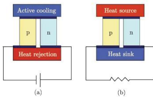
Рис. 8 Схематичне зображення термоелектричних модулів: (а) модуль охолодження, (б) модуль генерування електроенергії.
