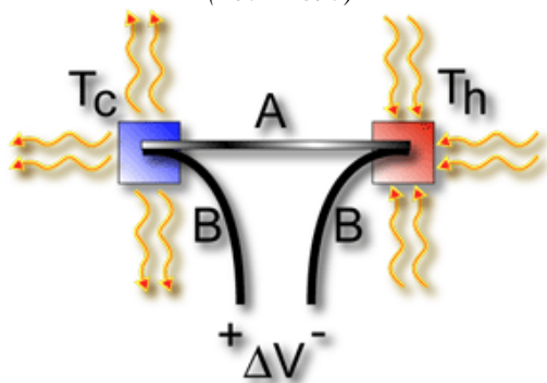
Рис. 4. Різниця потенціалів, V , яка виникає на розімкненому кінці кола, що складається із двох різномірних металів A і B , місця контакту яких знаходяться при різних температурах, прямо пропорційна різниці між гарячою та холодною температурами переходу T_h - T_c [7].
