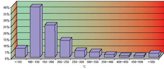
Рис. 1. Розподіл температур на поверхні промислових агрегатів [3].
