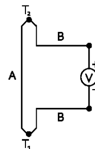
Рис. 3. а – демонстрація ефекту Зеебека (14 грудня 1820 року); б – принципова схема ефекту Зеебека.
