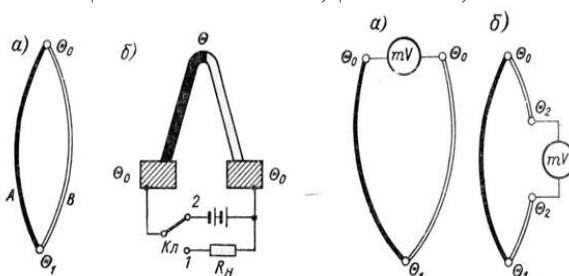
Рис. 5. Демонстрація термоелектричного охолодження (ефект Пельтьє, 1834 р.).
