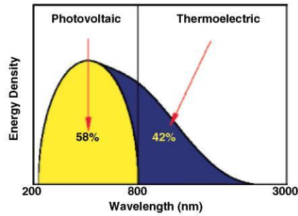
Рис. 2. Енергія сонячного випромінювання при 6000^{\circ}\text{C} для абсолютно чорної батареї із розділенням частин енергії в ультрафіолетовій та інфрачервоній областях спектру [5].
