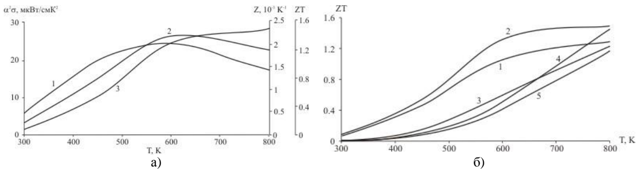
Рис. 2. Температурні залежності термоелектричної потужності a^2s – 1, розмірної Z – 2 та безрозмірної термоелектричної добротності ZT – 3 для x=0,25 (а) та безрозмірної термоелектричної добротності ZT (б) твердих розчинів PbTe_{1-x}Se_x складу x : 1 – 0,15; 2 – 0,25; 3 – 0,75; 4 – 0,85 та 5 – 0,95.
