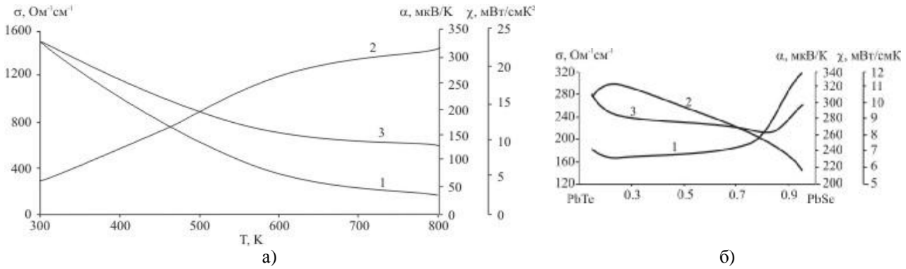
Рис. 1. Температурна залежність твердих розчинів PbTe_{1-x}Se_x складу x=0,25 (а) та залежність від складу при температурі 800 К (б) кінетичних параметрів: 1 – електропровідність \sigma , 2 – коефіцієнт термо-ЕРС \alpha , 3 – коефіцієнт теплопровідності \chi .
