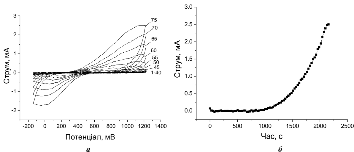
Рис. 4. ЦВА-криві AlNiCe-електрода: а – 1, 5, – 70, 75 цикли; б – кінетична крива формування анодного піку при E = \sim 1100 мВ.
