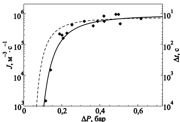
Рис. 7. Зависимость частоты нуклеации от избыточного давления при ОЦК–ГПУ переходе в растворе ^3\text{He} – ^4\text{He} с концентрацией 1,0% ^3\text{He} ( V_m = 20,98 см 3 /моль). Сплошная линия — расчет по формуле (7), штриховая линия — данные для переохлажденных отожженных образцов ОЦК фазы чистого ^4\text{He} при том же молярном объеме.
