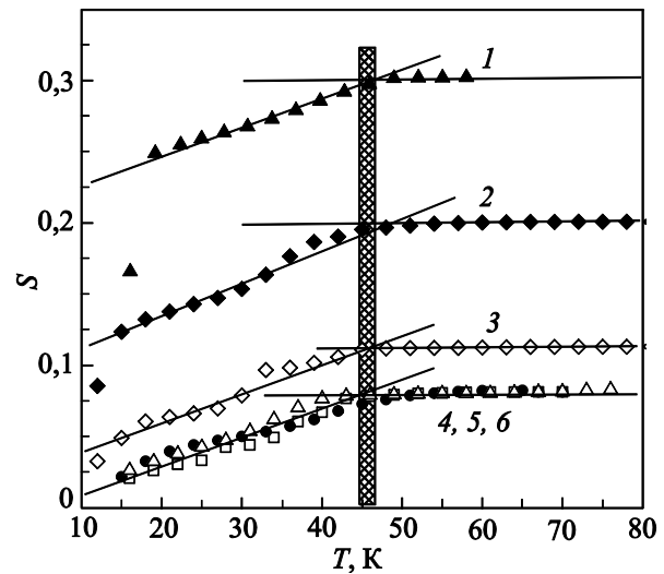
Рис. 2. Зависимости суммарной концентрации S(T) десорбированного водорода при нагреве образца от 12 К до температуры T для образцов, облученных в различных газовых средах: в дейтерии (1, \blacktriangle ), азоте (2, \blacklozenge ), кислороде (3, \diamond ), водороде (4, \Delta ), в вакууме (5, \bullet ), исходный необлученный образец (6, \square ).
