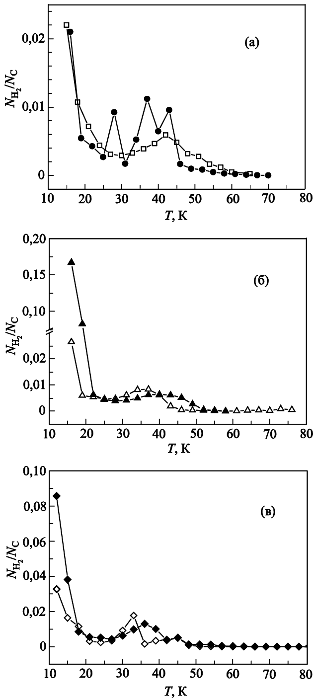
Рис. 1. Низкотемпературная десорбция молекулярного водорода из жгутов углеродных нанотрубок: (а) исходный необлученный образец ( \square ), образец, облученный в вакууме ( \bullet ); (б) образцы, облученные в водороде ( \Delta ) и дейтерии ( \blacktriangle ); (в) образцы, облученные в кислороде ( \diamond ) и азоте ( \blacklozenge ).
