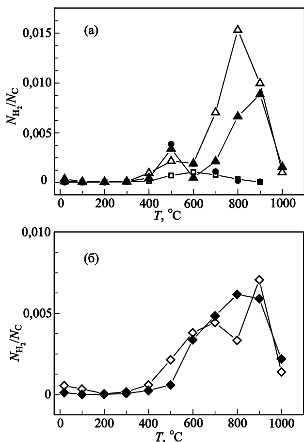
Рис. 7. Диаграммы высокотемпературной десорбции водорода из насыщенных водородом жгутов углеродных нанотрубок, облученных в различных условиях: (а) исходный необлученный образец (□), образцы, облученные в вакууме (●), водороде (Δ), дейтерии (▲); (б) образцы, облученные в кислороде (◇), азоте (◆).
