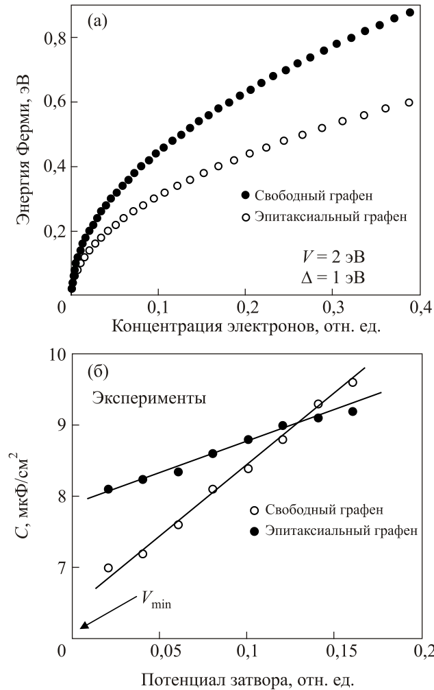
Рис. 6. Зависимость энергий Ферми свободного графена и ЭГ на полупроводниковой подложке от концентрации электронов (а); экспериментальные результаты зависимости квантовой емкости свободного [37] и ЭГ [38] (б). На рис. 6(б) нулевое значение потенциала затвора соответствует напряжению, при котором наблюдается минимум квантовой емкости.
