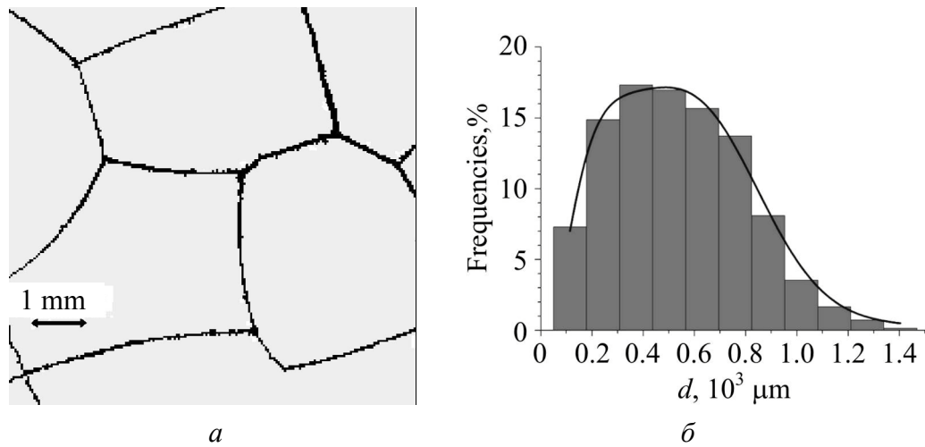
Рис. 1. Структура (а), гистограмма и оптимальная ФПР (б) зерен Nb–Ti-сплава
