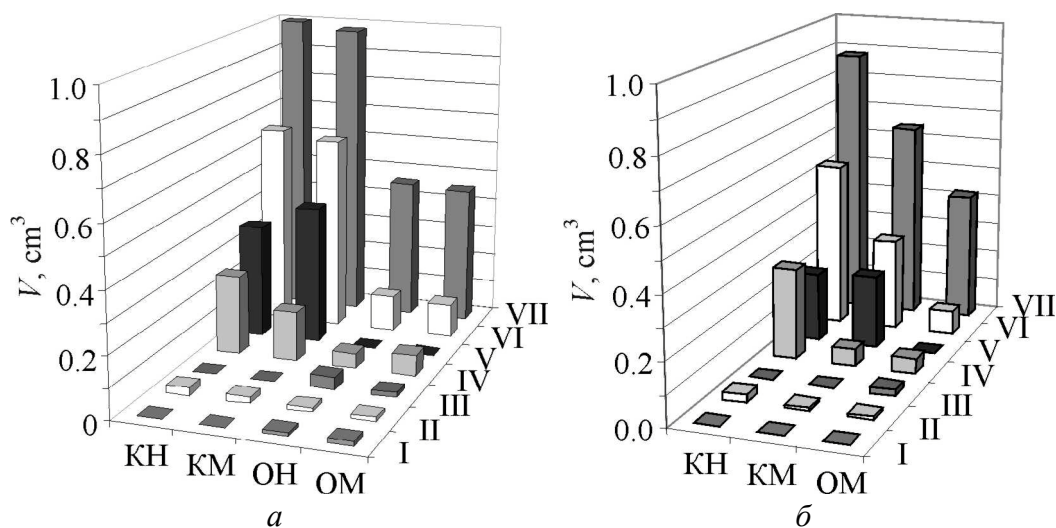
Рис. 2. Объемы поровых каналов в наноразмерных ксерогелях и пористых объектах из них: a – промывка ксерогелей водой, б – спиртом. Объем твердой фазы постоянен и равен 0.342 \text{ cm}^3 (на рисунке не приведен). КН и КМ – ксерогель немолотый и молотый; ОН и ОМ – спрессованный пористый объект из немолотого и молотого ксерогелей соответственно; I – каналы между «несвязанными» «первичными частицами», II – каналы между «первичными частицами» в агрегатах, III – каналы между «несвязанными» агрегатами, IV – каналы между агрегатами в агломератах и их фрагментах, V – каналы между агломератами, VI – все каналы, VII – суммарный объем (объемы твердой фазы и всех поровых каналов)
