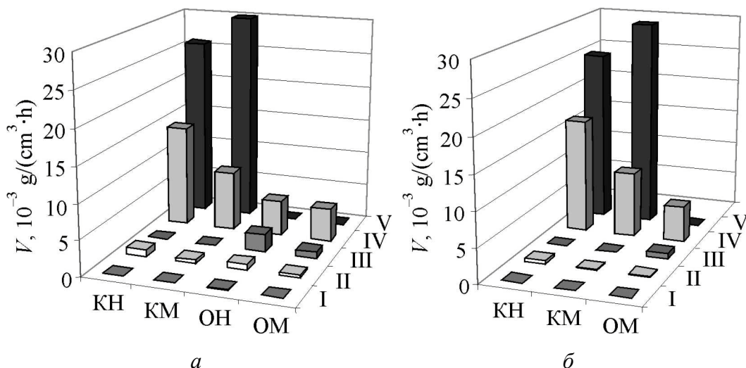
Рис. 3. Скорости испарения воды из поровых каналов в немолотых и молотых наноразмерных ксерогелях гидроокисей циркония и иттрия, промытых водой ( a ) и спиртом ( б ), и в пористых объектах, спрессованных из них. Обозначения те же, что на рис. 2
