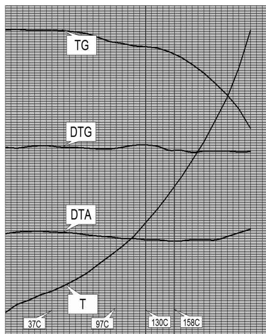
Рис. 2. Дериватограма СЕСК.
