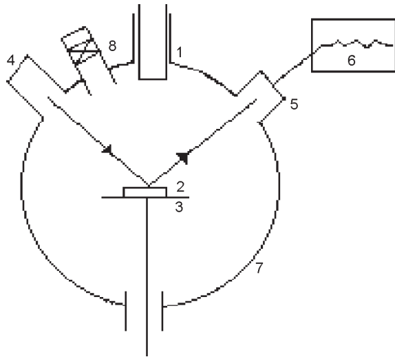
Рис. 1. Схема эксперимента: 1 – испаряемый металл; 2 – образец; 3 – подложкодержатель; 4 – лазер, ЛГ52-2; 5 – ФЭУ-85; 6 – потенциометр; 7 – вакуумная камера; 8 – газонатекаль.
