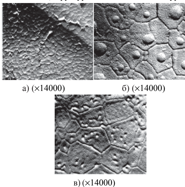
Рис. 12. Эрозионное разрушение TiN_x покрытия под воздействием воздушно-пылевого потока – а) и nc - TiN_x/a - SiN_y покрытие – в зоне отпечатка алмазного индентора – б).
