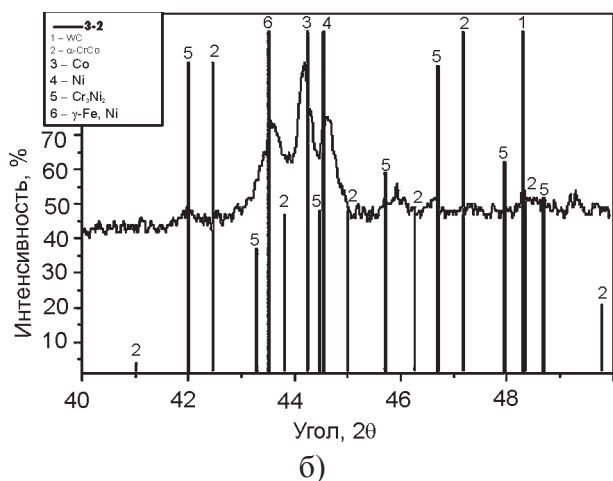
Рис. 1. Фрагменты дифрактограмм, полученных на образце с покрытием состава: Ni-Cr-B-Si-Fe/WC-Co со стороны покрытия – а) и после оплавления плазменной струей – б).
