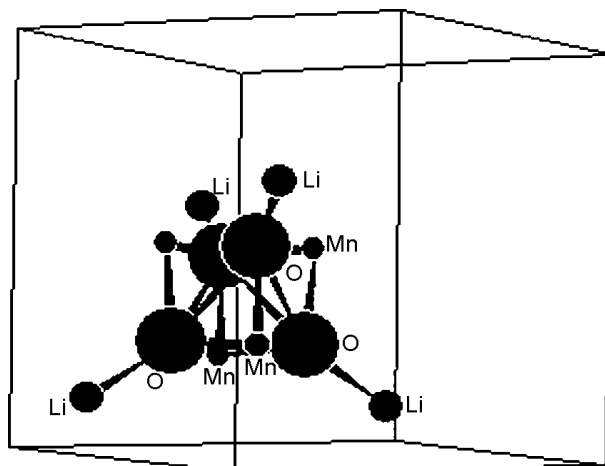
Рис. 4. Фрагмент кристалічної ґратки літій-марганцевої шпінелі.
