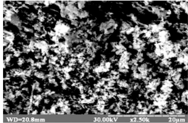
Рис. 2. Морфология поверхности GaAs после травления в электролите на основе \text{C}_2\text{H}_5\text{OH}:\text{HF} (1:1).
