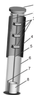
Рис. 1. Температурно-временные зависимости для кюветы с серой и для металлических прекурсоров в процессе их сульфуризации: а — образцы К 3.1, К 3.2, К 3.3; б — образец К 5.1. в — реактор для сульфуризации прекурсоров: 1 — клапан, дополнительно закрепленный пружиной; 2 — хромель-алюмелевая термопара для контроля температуры подложек; 3 — подложки; 4 — резистивный нагреватель; 5 — никелированный медный держатель; 6 — кварцевая труба; 7 — хромель-алюмелевая термопара для контроля температуры кюветы с серой; 8 — кювета с серой
