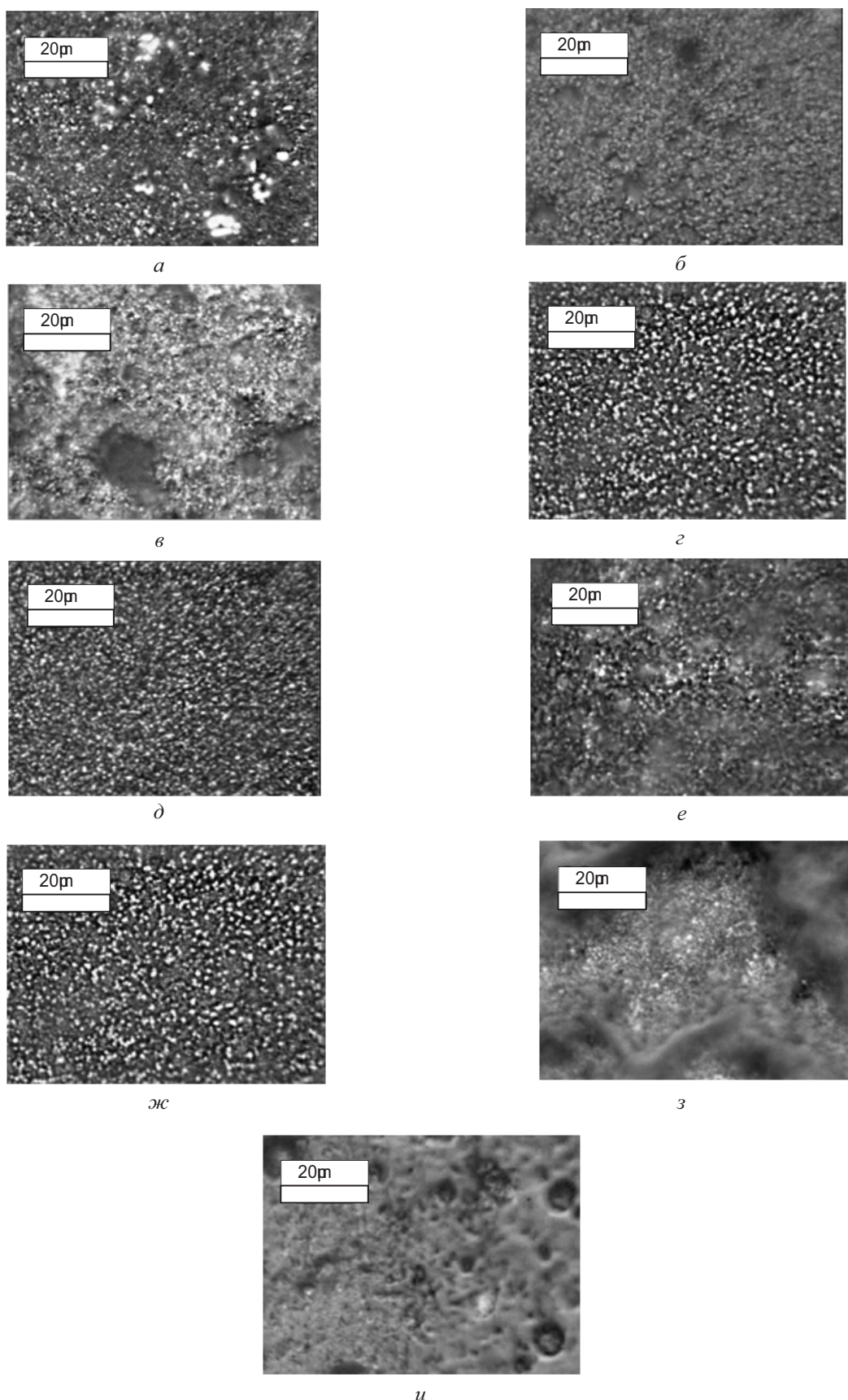
Рис. 2. Микрофотографии последовательно электроосажденных компонентов металлических прекурсоров: прекурсор образца К 3.1 ( a — слой Sn, б — слои Sn/Cu, в — слои Sn/Cu/Zn), прекурсор образца К 3.2 ( г — слой Cu, д — слои Cu/Sn, е — слои Cu/Sn/Zn), прекурсор образца К 3.3 ( ж — слой Cu, з — слои Cu/Zn, и — слои Cu/Zn/Sn)
