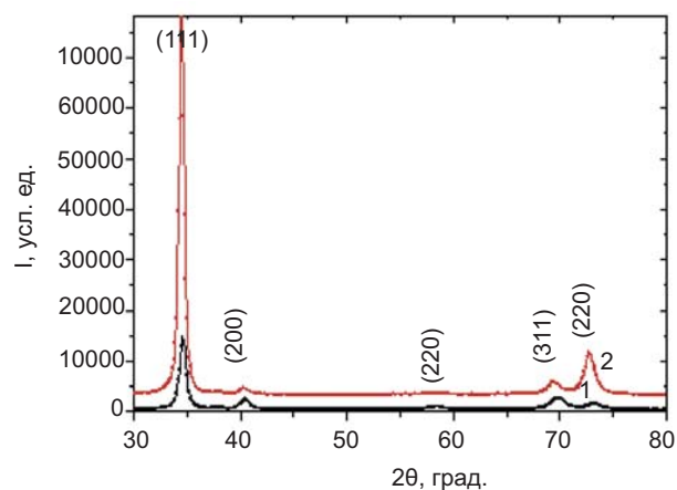
Рис. 6. Участки дифракционных спектров нитридных покрытий из высокоэнтропийного сплава Ti-Zr-Nb-V-Hf-Ta, полученных при U_n = -70 В (1) и -200 В (2)
