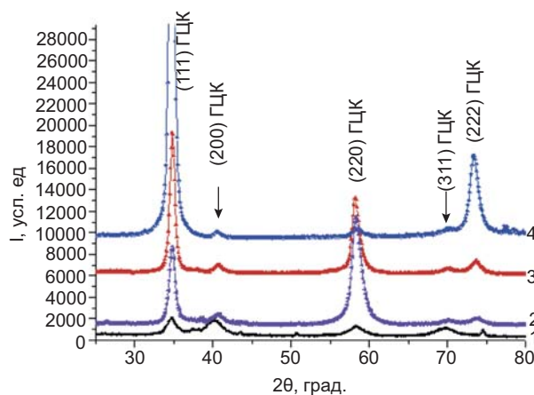
Рис. 1. Участки дифракционных спектров нитридных покрытий из высокоэнтропийного сплава Ti-Zr-Nb-V-Hf, полученных при U_{\text{н}} = -200 В и давлении азотной атмосферы ( P_{\text{N}_2} , Па): 1 — 0,04; 2 — 0,11; 3 — 0,27; 4 — 0,66
