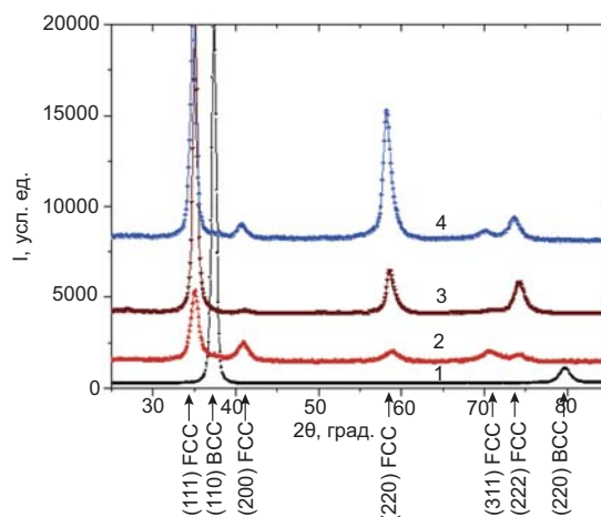
Рис. 2. Участки дифракционных спектров вакуумно-дуговых покрытий из высокоэнтропийного сплава Ti-Zr-Nb-V-Hf, полученных: 1 — при отсутствии азотной атмосферы ( H = 8,2 ГПа) и при P_{\text{N}_2} = 0,27 Па и U_{\text{н}} : 2 — -50 В ( H = 59 ГПа), 3 — -100 В ( H = 64 ГПа), 4 — -200 В ( H = 70 ГПа)
