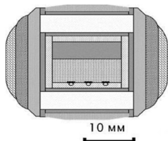
Рис. 1. Схематическое изображение ячейки высокого давления (а) и общий вид деталей сборки (б)
