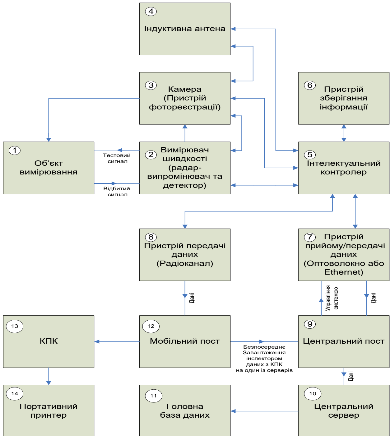
Рис. 3. Блок-схема комплексу
