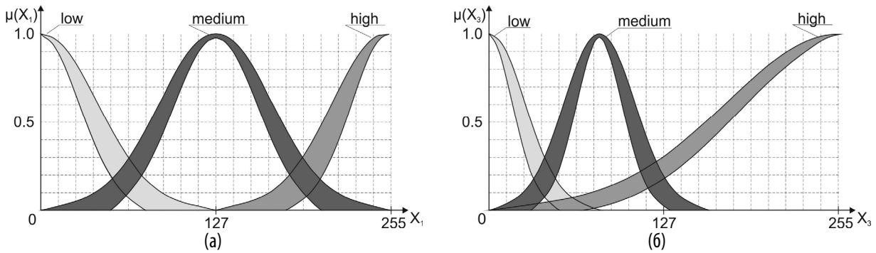
Рисунок 2 – Лінгвистическіе переменніе MG. (а) – лінгвистическіе переменніе A_1 ; (б) – лінгвистическіе переменніе A_3
