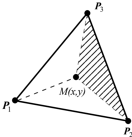
Рисунок 1 – Двумерный симплекс
