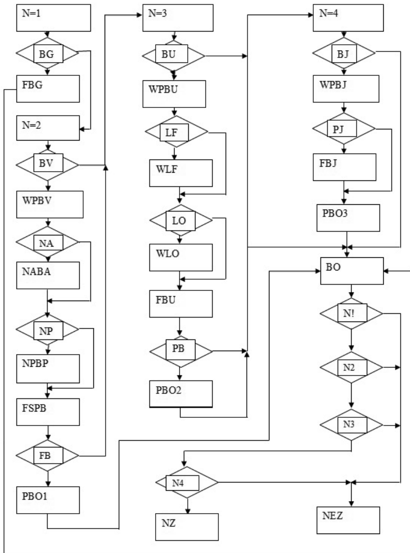
Рис. Функціональна схема
