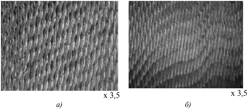
Рис. 1. Види вібраційних узоров на обробаній поверхні при продольному точенні. Умовля обробки: t = 2 мм; S = 0,15 мм/об.; D = 105,2 мм; матеріал деталі – Сталь 45 (HB163); матеріал інструмента – BK8; \varphi = 90^\circ ; \gamma = 0^\circ ; \alpha = 10^\circ ; \varphi_1 = 15^\circ ; \lambda = 0^\circ ; r = 0,2 мм: а) V = 82,6 м/мин.; б) V = 132,2 м/мин.
