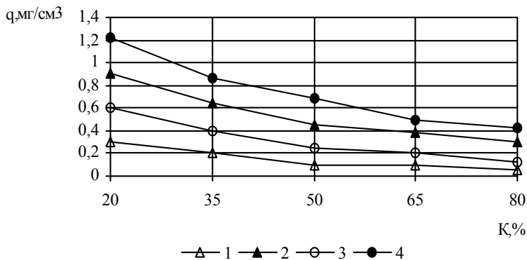
Рис. 3. Зависимость удельного расхода алмазного слоя «q» от концентрации алмазов «K» при зернистости Z = 2000/1600 мкм (1, 2), Z = 1000/800 мкм (3, 4) для карандашей из природных алмазов (1, 3) и алмазов типа СВ (2, 4) на связке М2-01 твердостью НВ180 при правке круга ПП1400х40х203 25А40СМ2К
