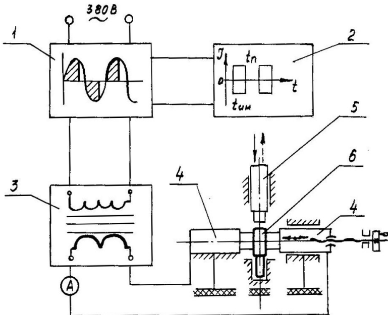
Рис. 1. Принципиальная схема установки для электроконтактного спекания алмазных карандашей:
