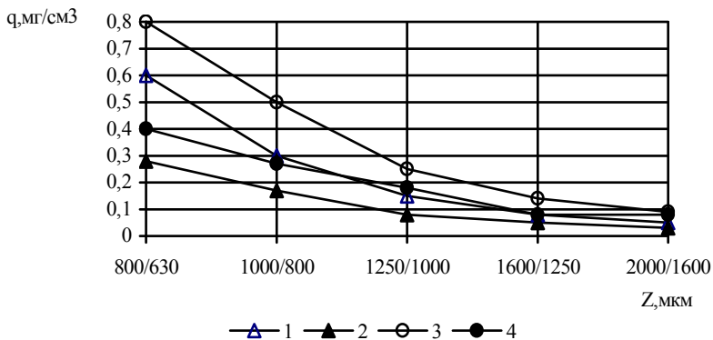
Рис. 4. Зависимость удельного расхода алмазного слоя «q» от зернистости алмазов «Z» при концентрации K = 80\% для карандашей из природных алмазов (1, 2) и алмазов типа СВ (3, 4) на связке М2-01 твердостью НВ180 (1, 3)
