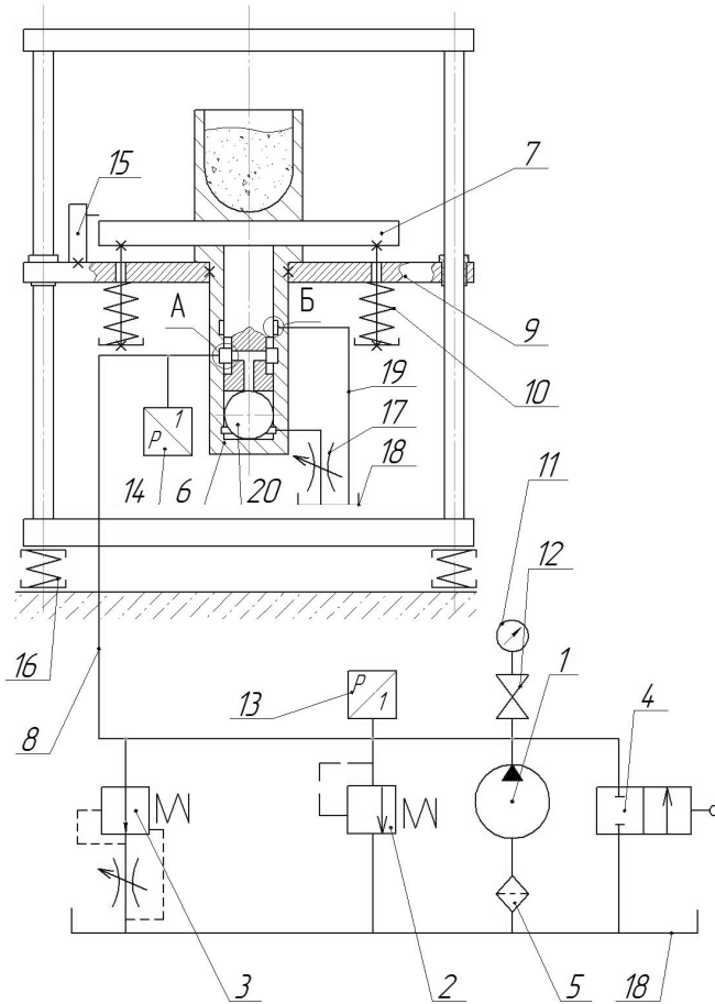
Рис. 3. Принципова гідрокінематична схема експериментальної віброустановки з одновісним накладанням вібрації
