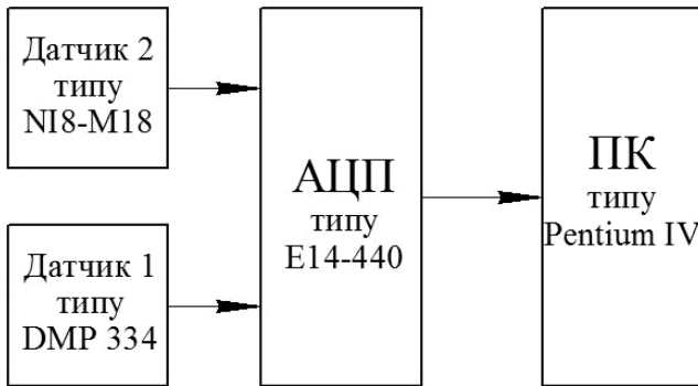
Рис. 2. Схема комплексу вимірювальної апаратури
