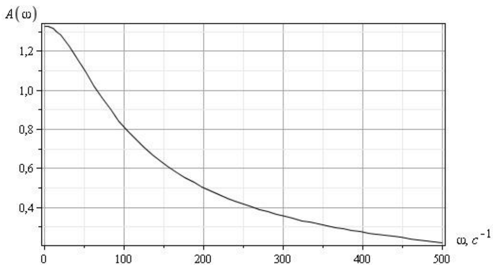
Рис. 3. Амплитудная частотная характеристика газогенератора
