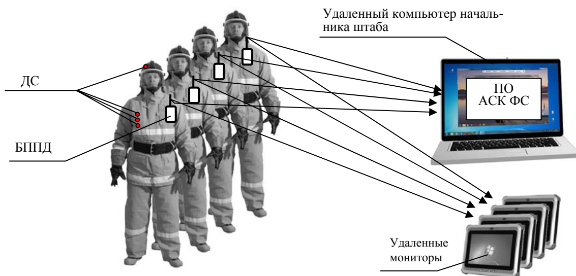
Рис. 1. Структурная схема АСКФС
