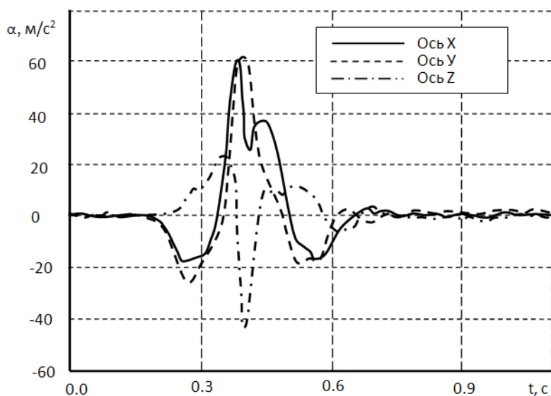
Рис. 4. Ускорения при имитации удара
