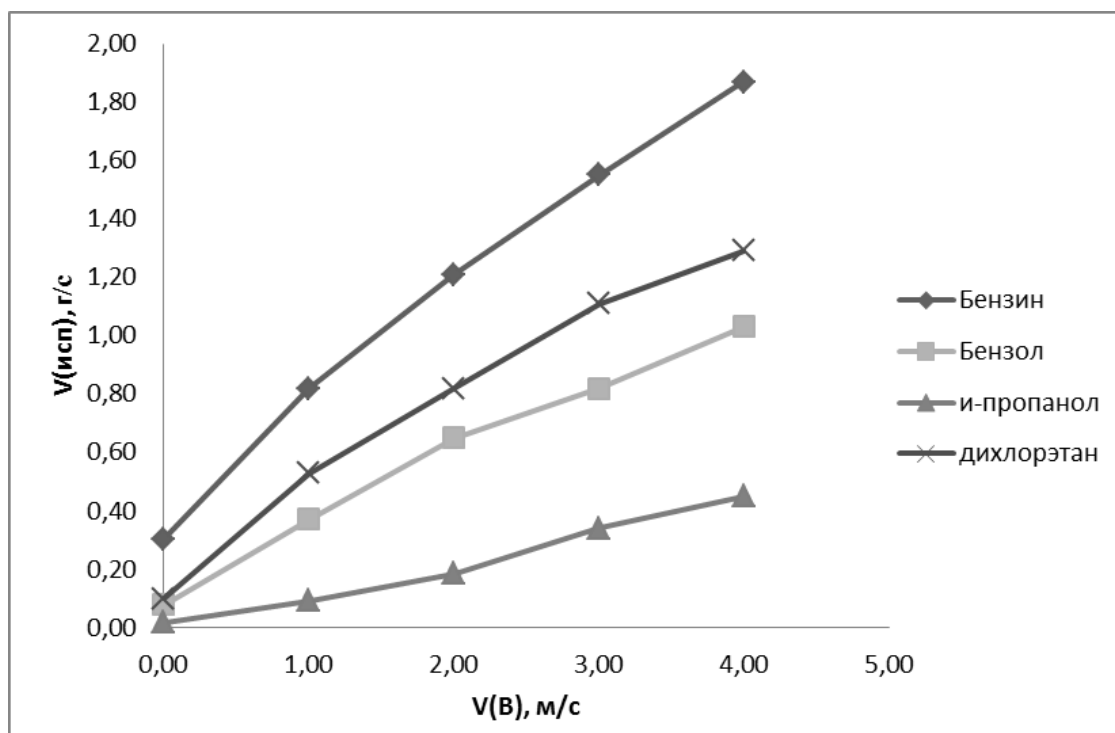
Рис. 1. Залежність швидкості випаровування рідин від інтенсивності вітрової навантаження
