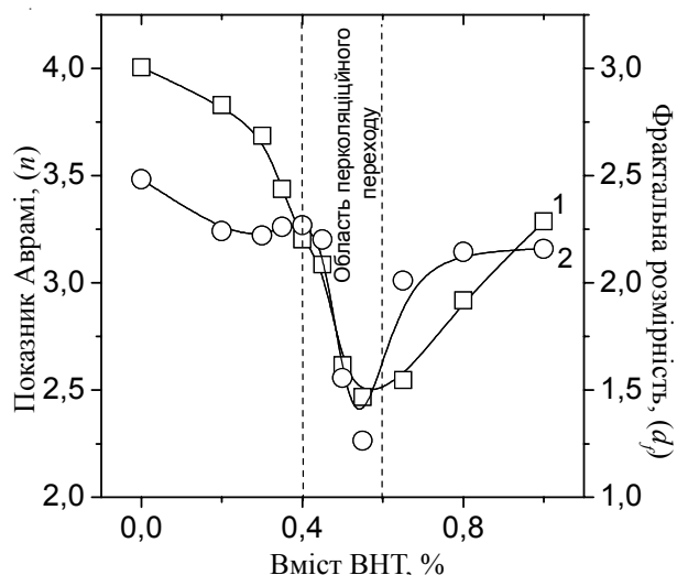
Рис. 4. Залежність показника Аврамі та фрактальної розмірності кристаліта, що росте, від вмісту ВНТ для нанонаповнених систем на основі ПЕО, за швидкостей охолодження: 2 (1) і 5 °C/хв (2)
