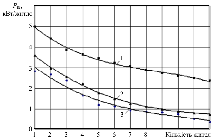
Рис. 2. Результат апроксимації значень розрахункової питомої електричної потужності залежно від кількості жител : 1 — за Державними будівельними нормами, 2 — за даними соціологічного опитування й теорією ймовірності, 3 — за даними АСКОЕ
