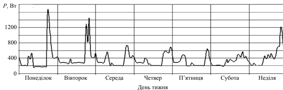
Рис. 1. Результат обробки інформації АСКОЕ щодо електричного навантаження житла першого виду першого рівня електрифікації 10-поверхового будинку протягом тижня
