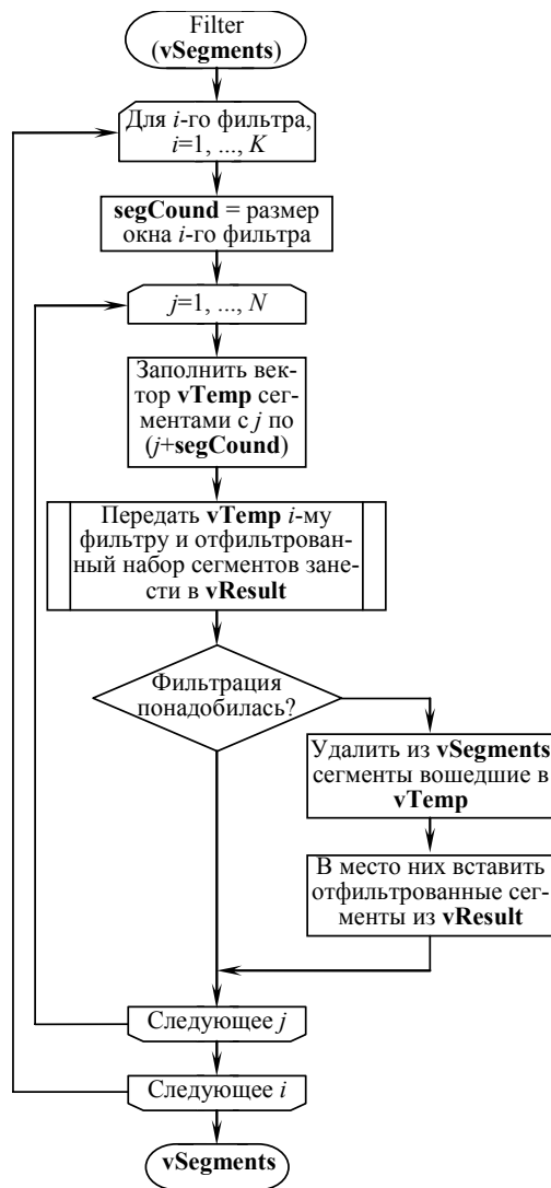
Рис. 2. Блок-схема алгоритма фильтрации набора сегментов
