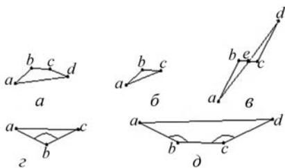
Рис. 3. Принцип работы алгоритма фильтрации. Предполагается, что все длины сегментов меньше заданного порогового значения ( a...в ) и все обозначенные углы меньше порогового значения ( г, д )
