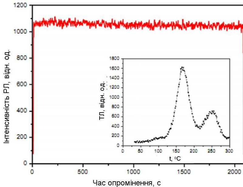
Рис. 3. Залежність інтенсивності радіюлюмінесценції монокристалічного зразка ТБЛ: Аg від часу опромінення при потужності дози 0.5 мГр/с. На вкладинці – крива термовисвічування після опромінення (доза 1 Гр) впродовж 2000 с.
