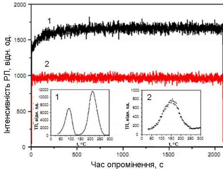
Рис. 2. Залежність інтенсивності радіюлюмінесценції зразків ТБЛ: Мп від часу опромінення при потужності дози 0,5 мГр/с. (1 – монокристал, 2 – скло). На вкладинці – криві термовисвічування монокристалічних (1) і склоподібних (2) зразків після опромінення (доза 1 Гр) впродовж 2000 с.
