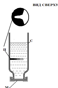
Рис. 34. Приспособление для вскрытия и отбора газовой фазы в ампулах
