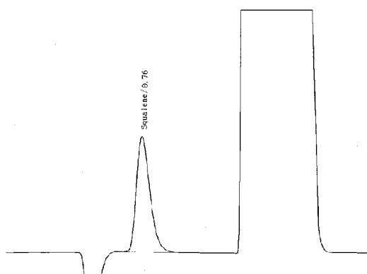
Рис. 62. Хроматограмма испытуемого раствора масла амаранта, полученная в режиме переключение направления подвижной фазы
