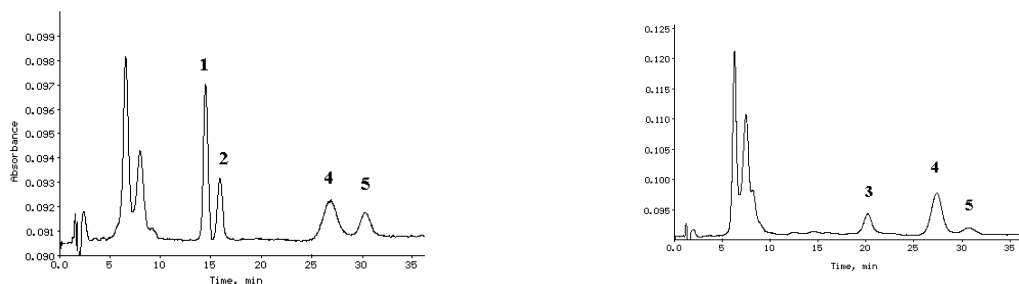
Рис. 50. МЖХ хроматограммы экстрактов растительного лекарственного сырья. Сверху - вниз: экстракт коры крушины, экстракт корней ревеня, экстракт корневищ щавеля. 1 – реин; 2 – эмодин; 3 – реум-эмодин; 4 – хризифанол; 5 – фисцион
