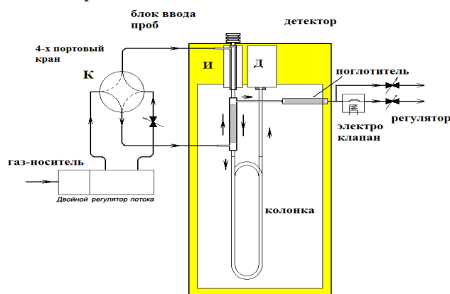
Рис. 52. Схема хроматографической системы, предназначенная для непосредственного определения сквалена в жирных маслах
