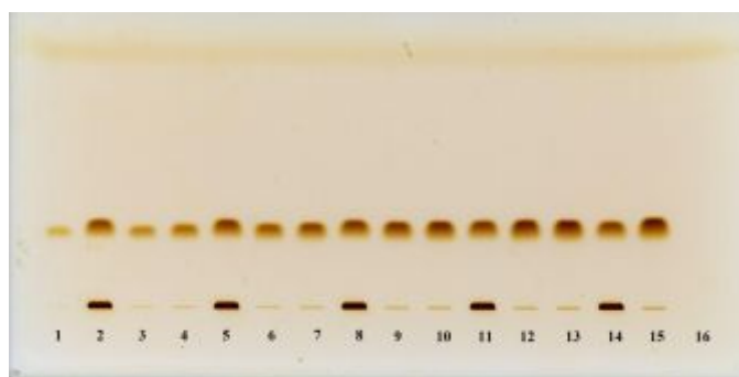
Рис. 73. Изображение пластинки с хроматограммами испытуемого раствора масла амаранта (2, 5, 8, 11 и 14), растворов сравнения сквалена (1, 3, 4, 6, 7, 9, 10, 12, 13, 15) и растворителя (16)
