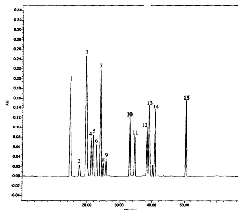
Рис. 18. Хроматограмма раствора РСО для анализа препарата Аминол. Порядок выхода пиков 2,4-динитрофенилпроизводных аминокислот: 1 - 2,4-динитрофторбензол, 2 - гистидина гидрохлорид, 3- глицин, 4- метионина сульфон, 5 - метионин, 6 - аргинина гидрохлорид, 7 - лизина гидрохлорид, 8 - аланин, 9 - пролин, 10 - треонин, 11 - валин, 12 - изолейцин, 13 – лейцин, 14 - фенилаланин, 15 - триптофан
