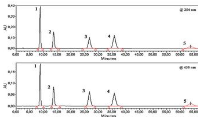
Рис. 48. ВЭЖХ хроматограмма разделения алоэ-эмодина (1), реина (2), эмодина (3), хризофанол (4) и фисиона (5)
