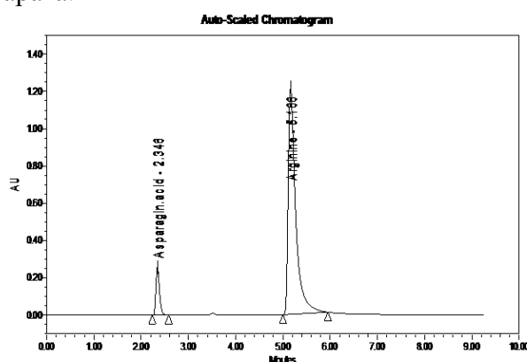
Рис. 24. Типичная хроматограмма раствора стандартного образца (PCO) аргинина и кислоты аспарагиновой методом ВЭЖХ
