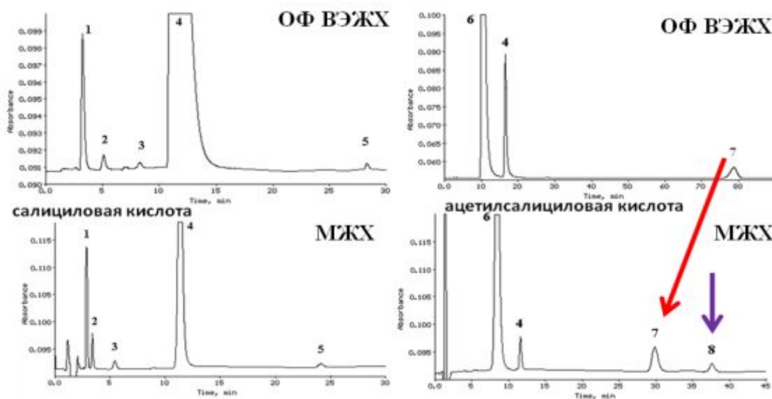
Рис. 44. Хроматограммы определения примесей в субстанциях салициловой кислоты (слева) и ацетилсалициловой кислоты (справа) двумя методами. 1 – 4-гидроксibenзойная кислота; 2– 4-гидроксиизофталева́я кислота; 3 – фенол; 4 – салициловая кислота; 5 – салицилсалициловая кислота; 6 – ацетилсалициловая кислота; 7 – ацетилсалицилсалициловая кислота; 8 – ацетилсалициловый ангидрид
