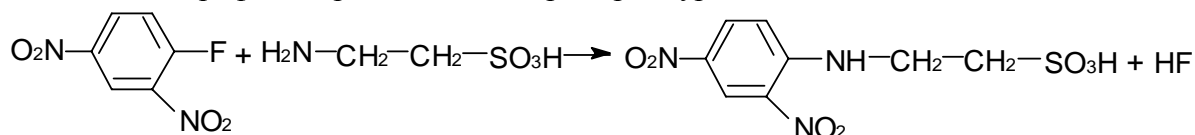
Рис. 20. Схема получения 2,4-динитрофенилпроизводного Таурина
