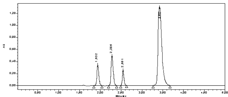
Рис. 29. Хроматограмма исследуемого раствора геля Димецин: 1 - L-лизина эсцинат; 2 – ДМСО; 3 – нипагин, 4 - диклофенак натрия
