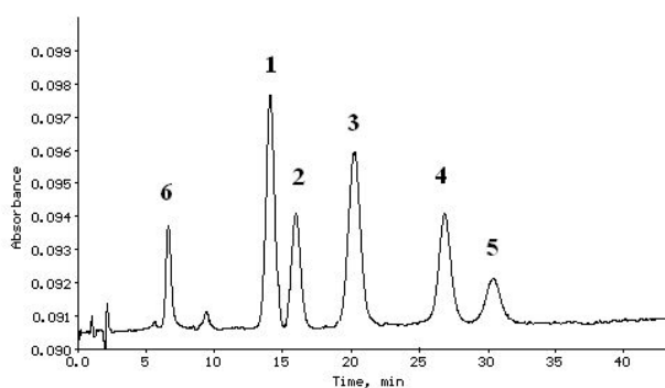
Рис. 49. МЖХ хроматограмма модельной смеси антрахинонов. 1 – реин; 2 – эмодин; 3 – реум-эмодин; 4 – хризофанол; 5 – фисион; 6 – сумма франгулинов и глюкофрангулинов
