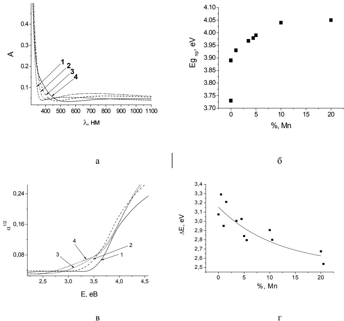
Рис. 3. а) Спектри поглинання плівок 1 – \text{TiO}_2 , 2 – 1% \text{Mn}/\text{TiO}_2 , 3 – 10% \text{Mn}/\text{TiO}_2 , 4 – 20% \text{Mn}/\text{TiO}_2 ; б) Залежність ширини забороненої зони для прямих переходів електрона з валентної зони у зону провідності від концентрації допанта для плівок \text{Mn}/\text{TiO}_2 , в) залежність коефіцієнта поглинання від енергії падаючого випромінювання \alpha^{1/2}=f(E) для плівок 1 – \text{TiO}_2 , 2 – 1% \text{Mn}/\text{TiO}_2 , 3 – 10% \text{Mn}/\text{TiO}_2 , 4 – 20% \text{Mn}/\text{TiO}_2 ; г) залежність ширини забороненої зони плівок від концентрації допанта.
