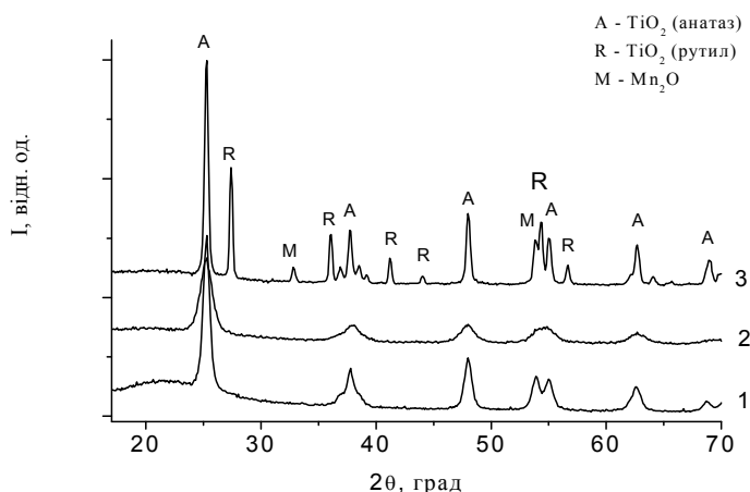
Рис. 2. Рентгенограми порошоків \text{TiO}_2 (1), \text{Mn}/\text{TiO}_2 , прожарених при 450 (2) і 650 \text{ }^\circ\text{C} (3).
