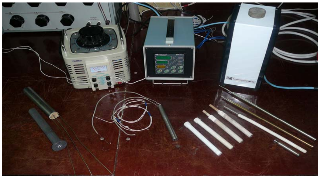
Рис. 1. Экспериментальная установка для определения теплофизических характеристик строительных материалов
